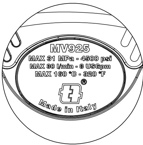
DETTAGLIO-DETAIL A
